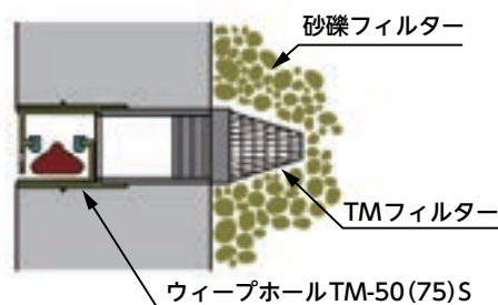
側壁用
